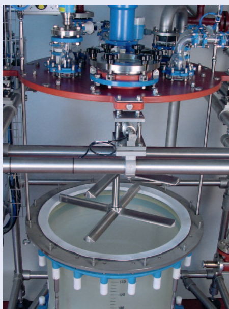
150 l solidphase reactor with filter, stirrer and load cells Solidphase-Reaktor mit Filter, Rührer und Wägezellen
