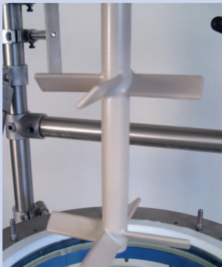
Various stirrer shapes and materials Verschiedene Rührerformen und Materialien
